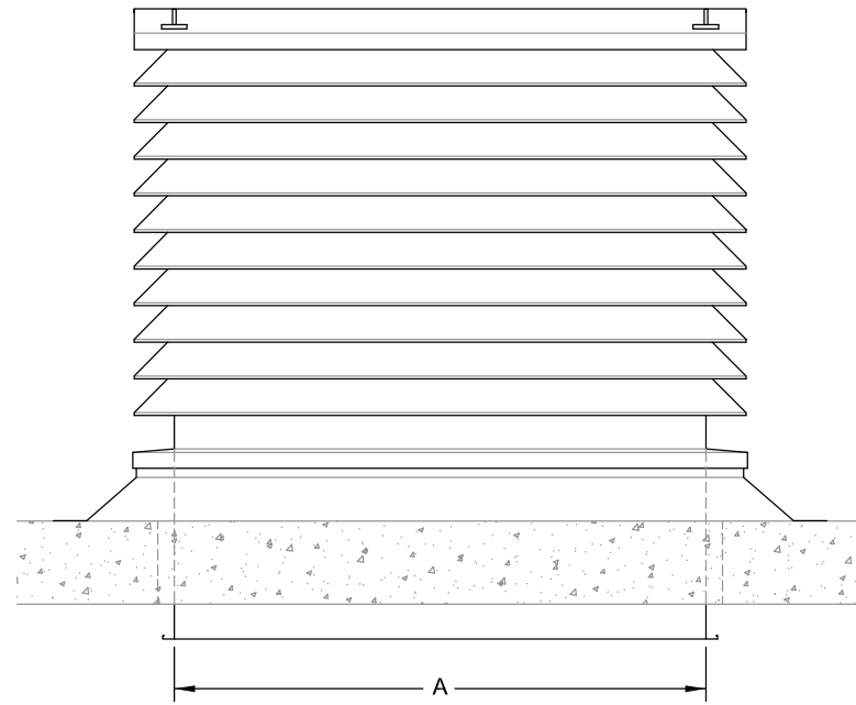
zij aanzicht schoepenkap
