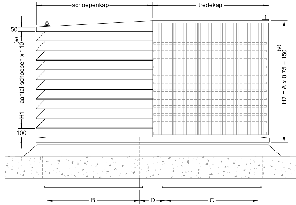
vooraanzicht
