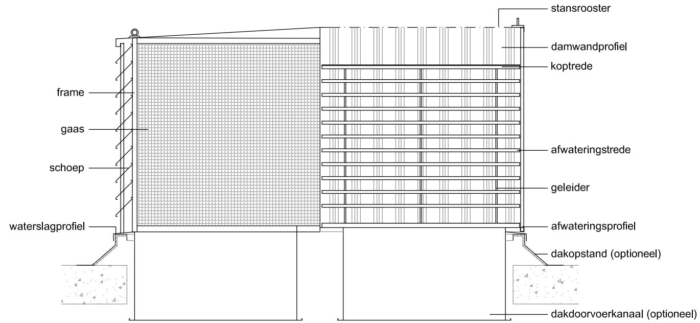
doorsnede
